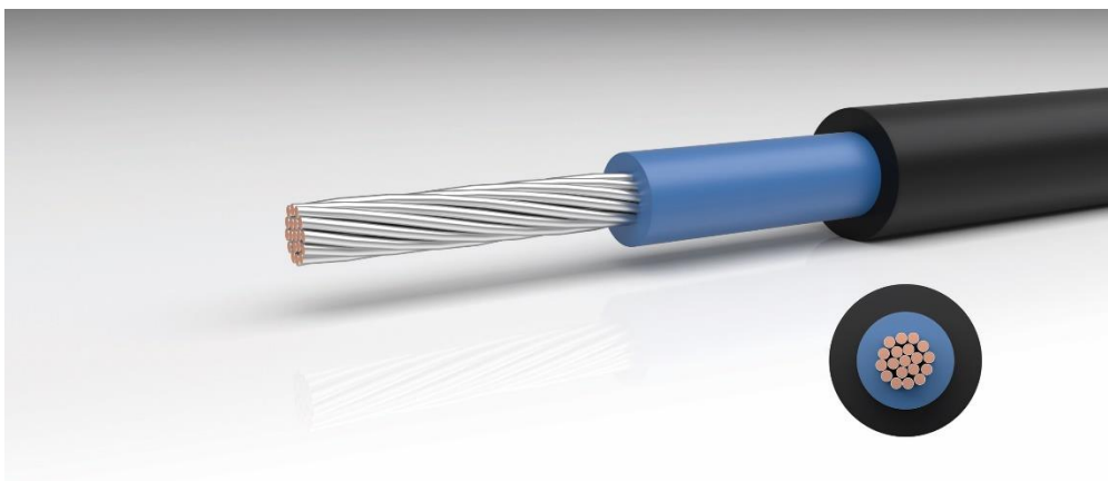
Obrázok A.22 – Vzhľad kábla EFK SOLAR a EFK SOLAR-80
