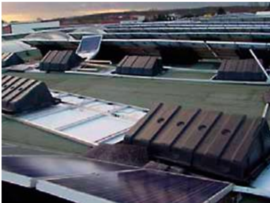
Obrázok 1 – Dôsledky nesprávneho upevnenia FVE na streche po búrke
