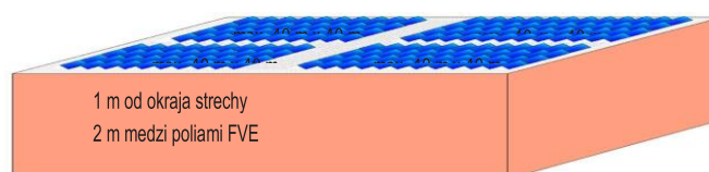
Obrázok 9 – Príklad inštalácie šikmých modulov na plochú strechu bez požiarného oddelenia
