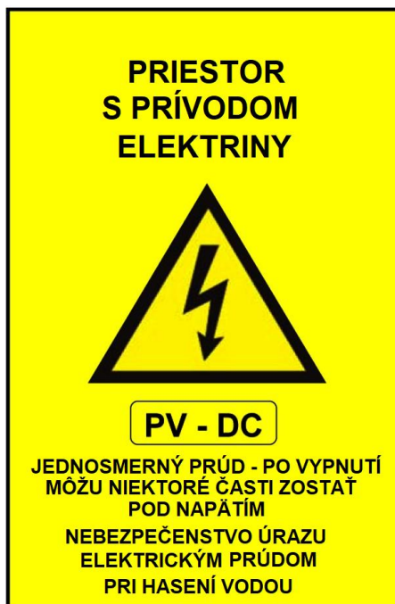
Obrázok 19 – Označenie priestoru s káblami na jednosmerný prúd alebo striedačmi
