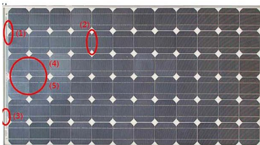
Obrázok A.5 – Miesta v moduloch, kde môže dôjsť k poruchám
