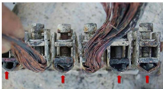
Obrázok A.27 – Stav elektrických spojov po požiari
