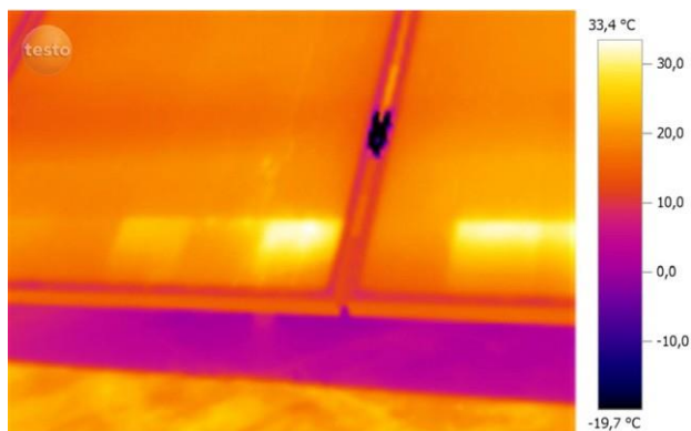
Obrázok A.6 – Zobrazenie horúcich bodov na termovíznej kamere
