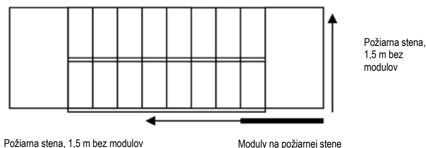
Obrázok 26 – Schematický pôdorys znázorňujúci požiadavky na inštaláciu FVE vedľa chráneného schodiska
