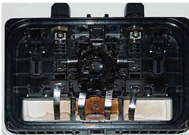
Obrázok A.13 – Dôsledky elektrického oblúka vo vnútri prípojného portu FV modulu
