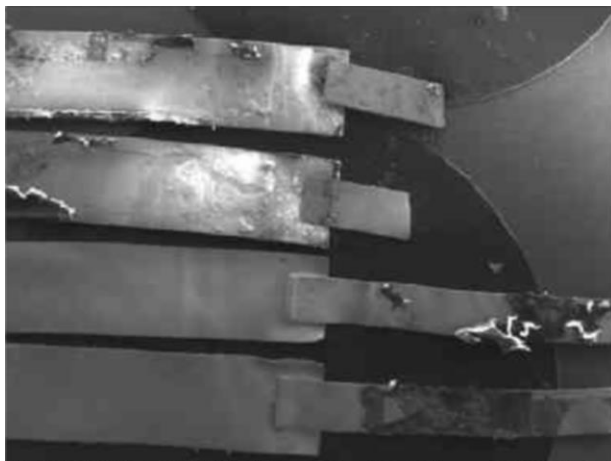
Obrázok A.9 – Vodiče prípojnice vo vnútri modulu – zvýšený ohmický odpor a prehrievanie
