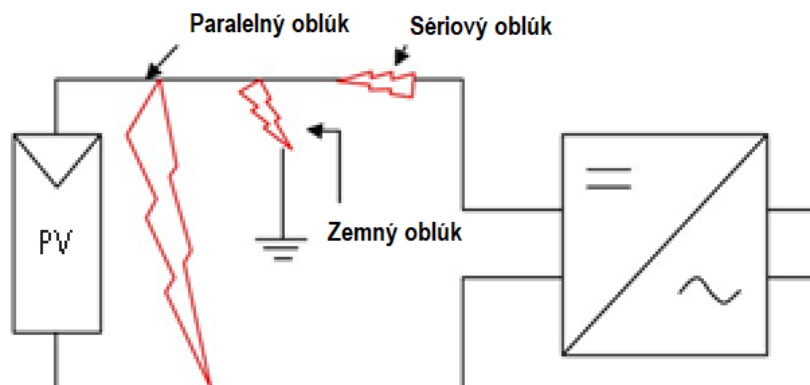
Obrázok A.2 – Schematický príklad elektrických oblúkov
