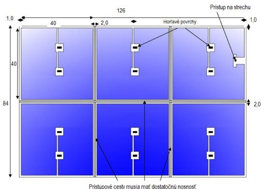
Obrázok 10 – Príklad šiestich poľí modulov na plochej streche s primeraným prístupom pre zásah
