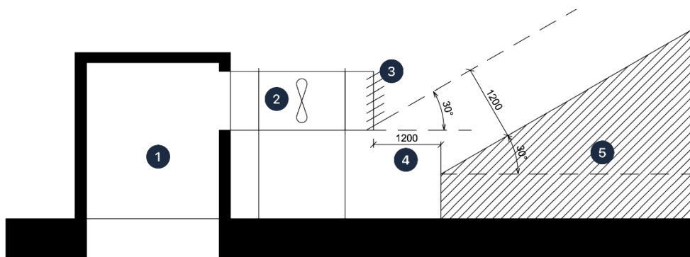
Obrázok 3b – Príklad správnej inštalácie ZOTSH na streche s FVE v horizontálnej polohe
