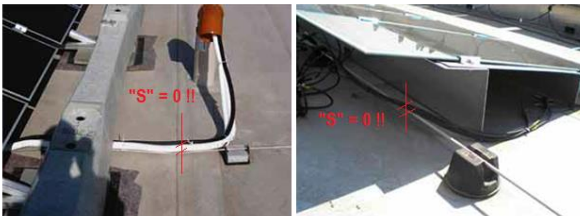
Obrázok A.28 – Dva príklady nedostatočnej vzdialenosti „s“ zvodu bleskozvodu od kábla FVE
