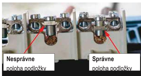
Obrázok 16 – Príklad vhodného a nevhodného spojenia s dôsledkami
