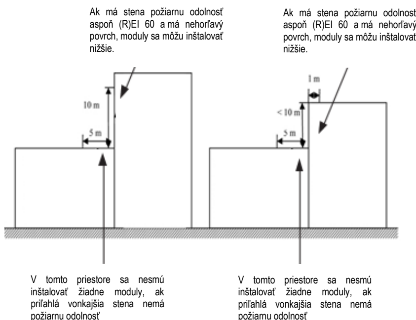
Obrázok 25 – Schematický prierez budovy s uvedením požiadaviek na požiaru odolnosť
