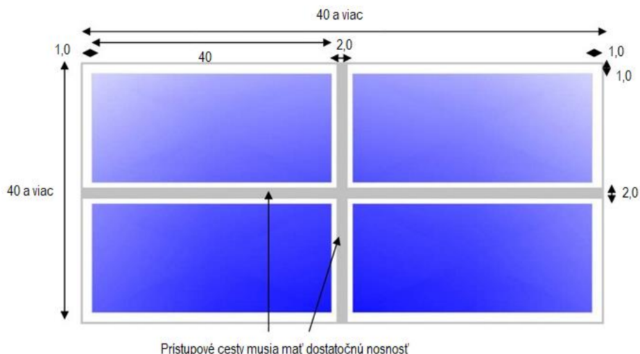
Obrázok 11 – Príklad štyroch polí modulov na plochej streche s primeraným prístupom pre zásah
