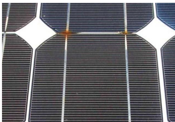
Obrázok A.7 – Účinky prehriatia viditeľné na povrchu modulu
