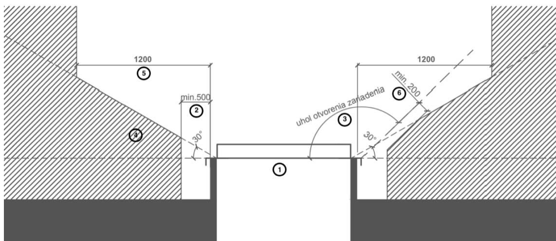
Obrázok 3a – Príklad správnej inštalácie ZOTSH na streche s FVE vo vertikálnej polohe
