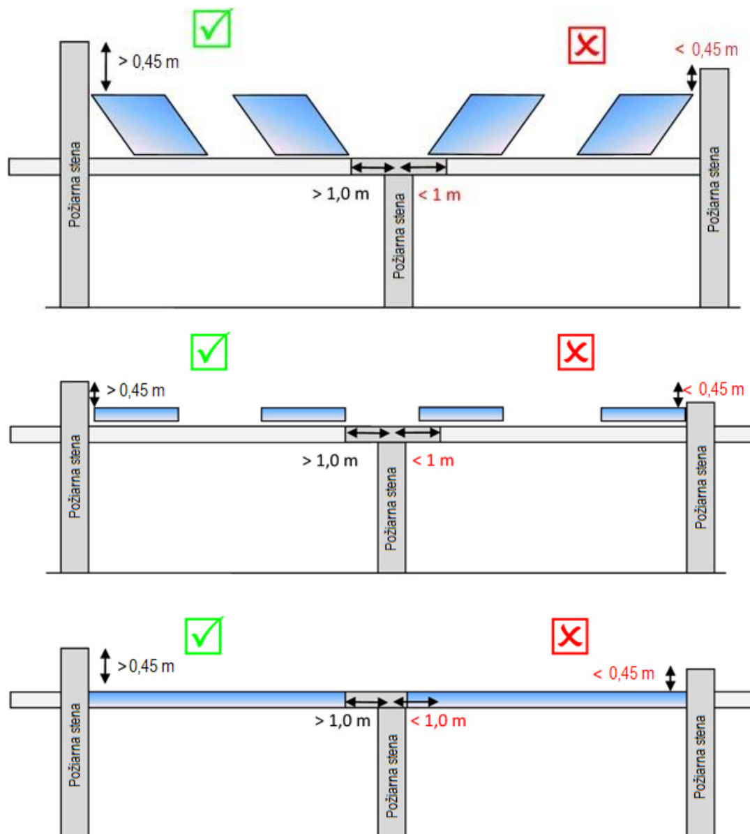
Obrázok 4 – Príklady správneho a nesprávneho umiestnenia modulov
