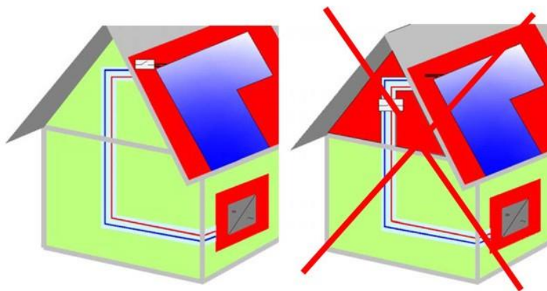
Obrázok 15 – Príklad správneho a nesprávneho umiestnenia oddeľovacích prvkov
