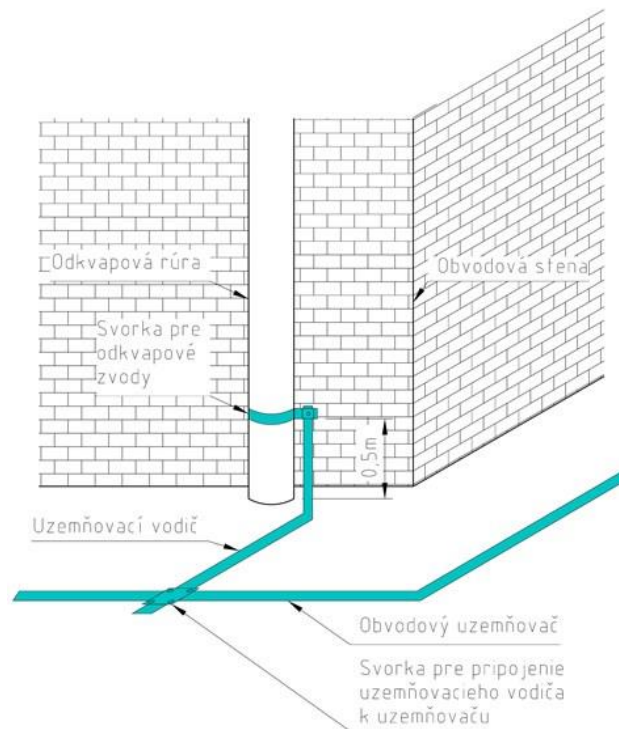
Obrázok 8 – Príklad uzemnenia odkvapovej zvodovej rúry bez blízko vedeného zvodu
