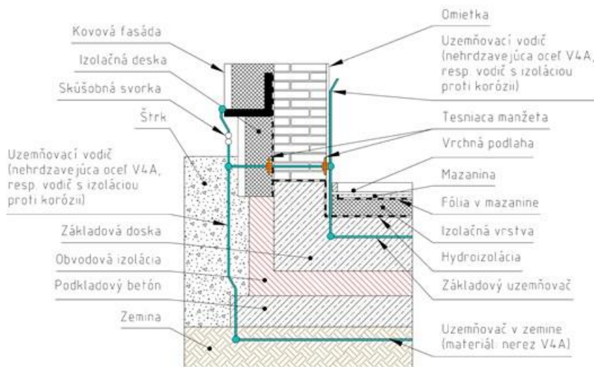
Obrázok 14 – Príklad vyvedenia uzemňovacieho vodiča z obvodového uzemňovača typu B
