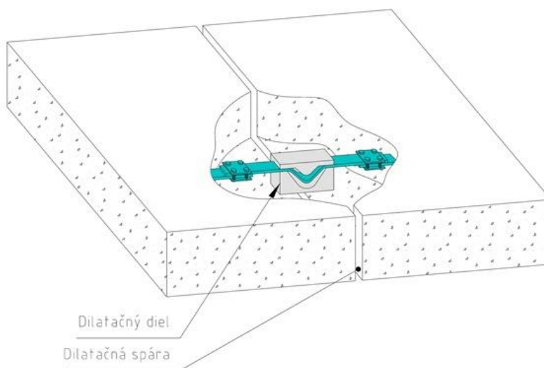
Obrázok 21 – Príklad vodorovnej dilatácie uzemnenia v základových doskách
