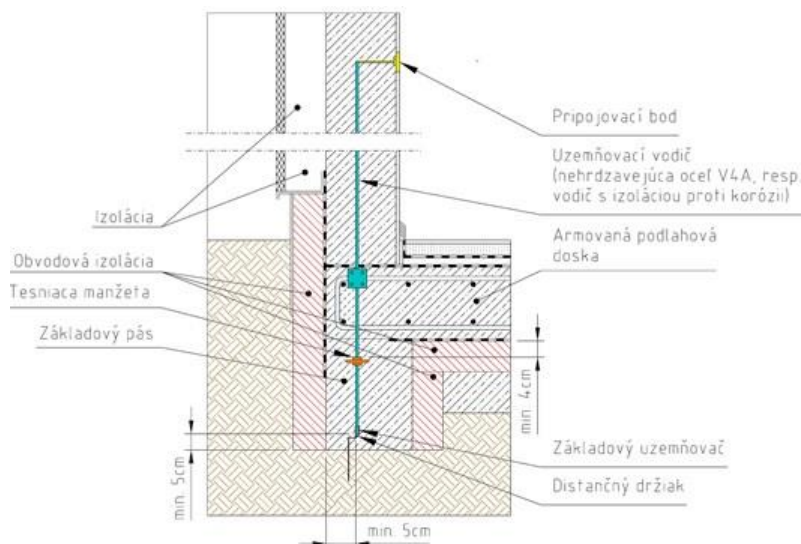
Obrázok 13 – Príklad vyvedenia uzemňovacieho vodiča zo základového uzemňovača typu B
