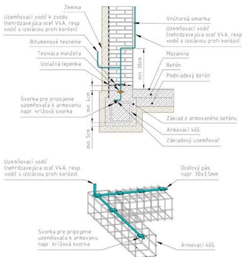
Obrázok 11 – Príklad vyvedenia uzemňovacieho vodiča zo základového uzemňovača typu B č.2
