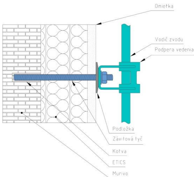
Obrázok 7 – Upevnenie podpory vedenia zvodu cez ETICS do stavebnej konštrukcie kotvou
