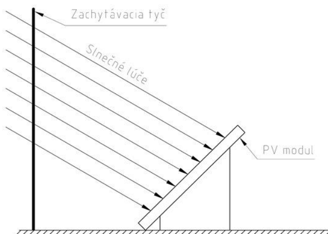
Obrázok 1 – Zatiernenie PV modulu zachytávacou tyčou
