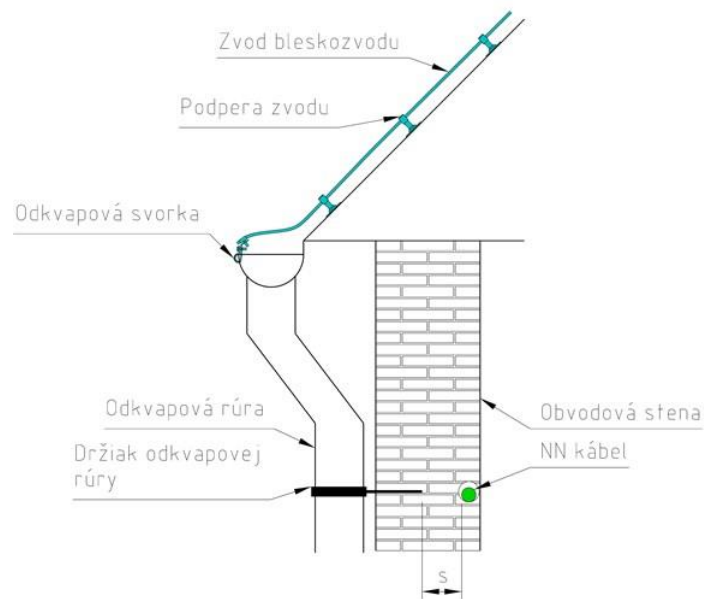
Obrázok 9 – Príklad dostatočnej vzdialenosti „s“
