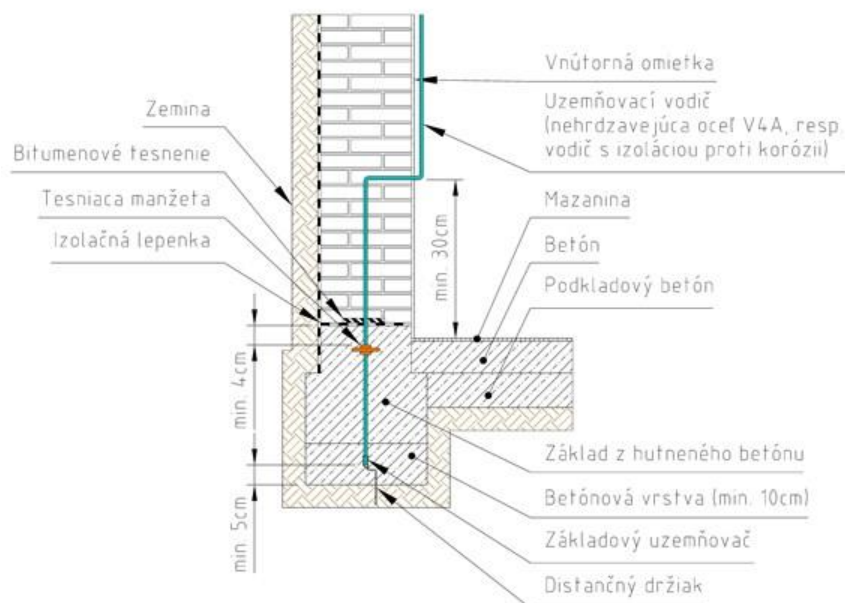
Obrázok 10 – Príklad vyvedenia uzemňovacieho vodiča zo základového uzemňovača typu B č.1
