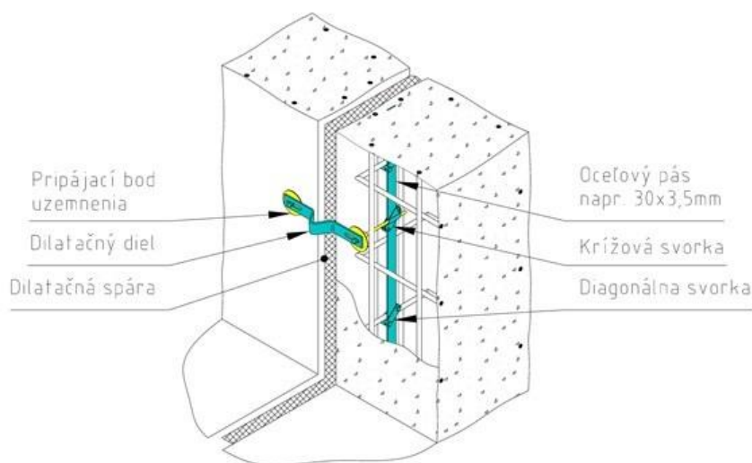
Obrázok 19 – Príklad zvislej dilatácie uzemnenia v obvodových konštrukciách
