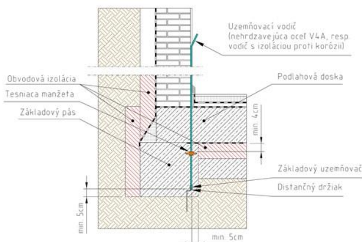
Obrázok 12 – Príklad uloženia základového uzemňovača typu B
