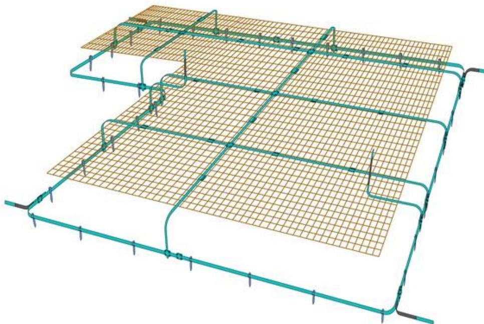
Obrázok 20 – Základový uzemňovač so sieťou vyrovnania potenciálov
