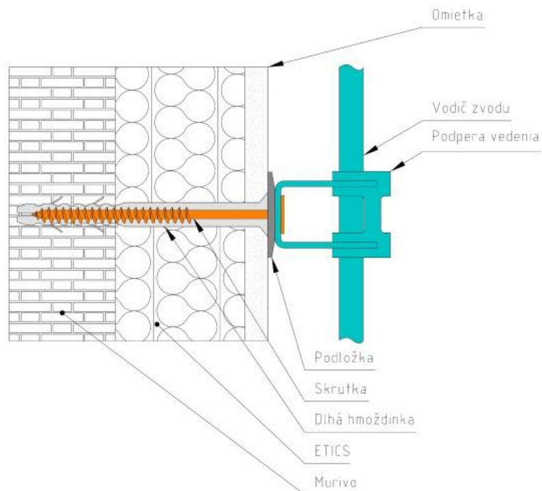
Obrázok 6 – Upevnenie podpory vedenia zvodu cez ETICS do stavebnej konštrukcie hmoždinkou
